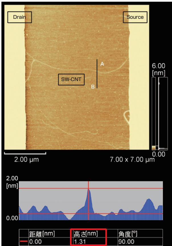
形状像と線分A-Bでの形状プロフィール Topographic image and Profile of topograph
