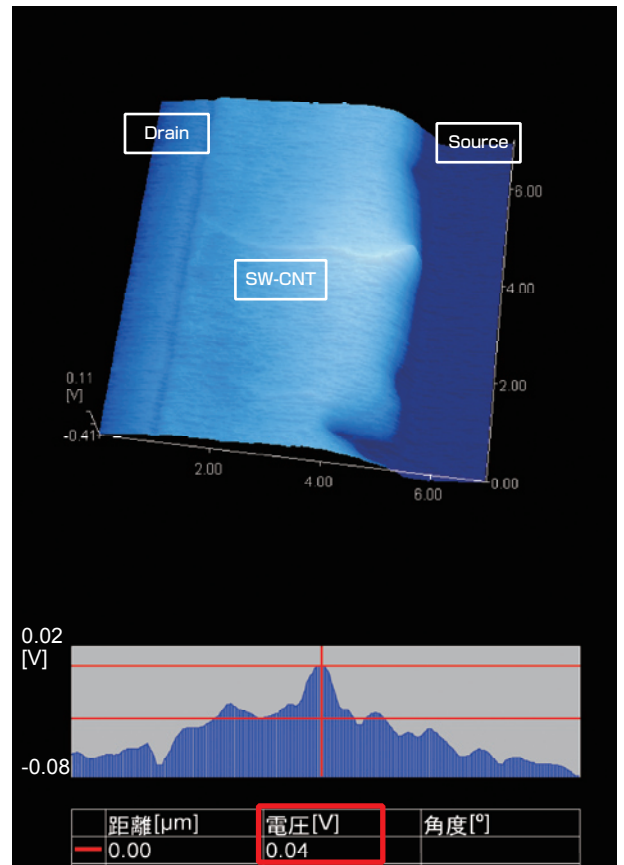
電位像と線分A-Bでの電位プロフィール Electric potential image and Profile of electric potential
