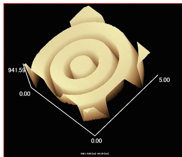
AFM像 (2万倍 : 5 \mu m × 5 \mu m)
