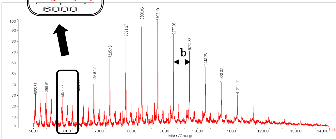
MALDI-TOFMS (AXIMA-CFR) スペクトル
